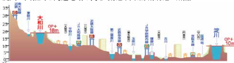
淀川・大和川と周辺地域の高さ(府道中央環状線付近の断面)
